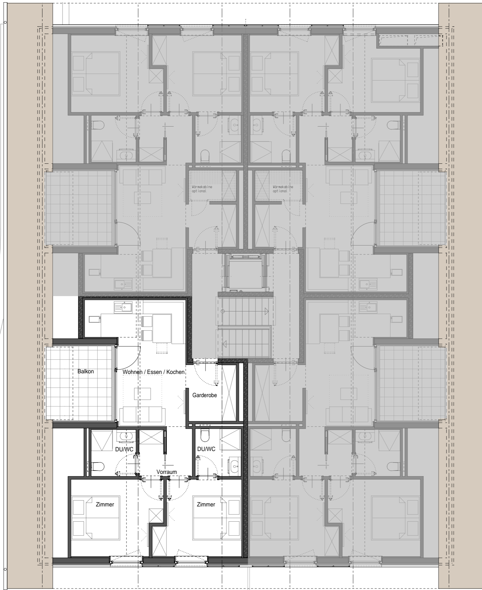
Grundriss Haus 3 E+4 M 1:100
